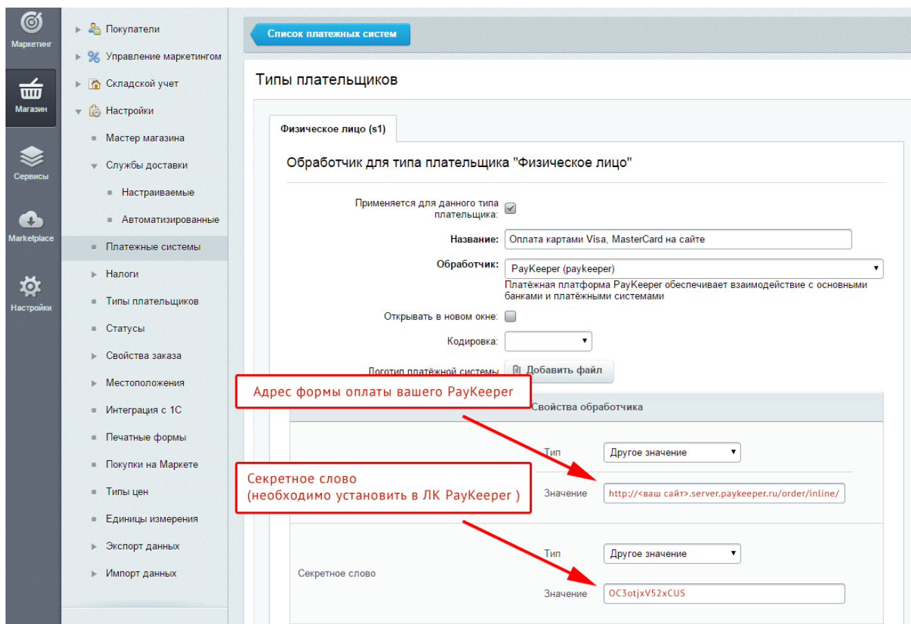
Рисунок 3. Настройка системы для типа плательщика.
