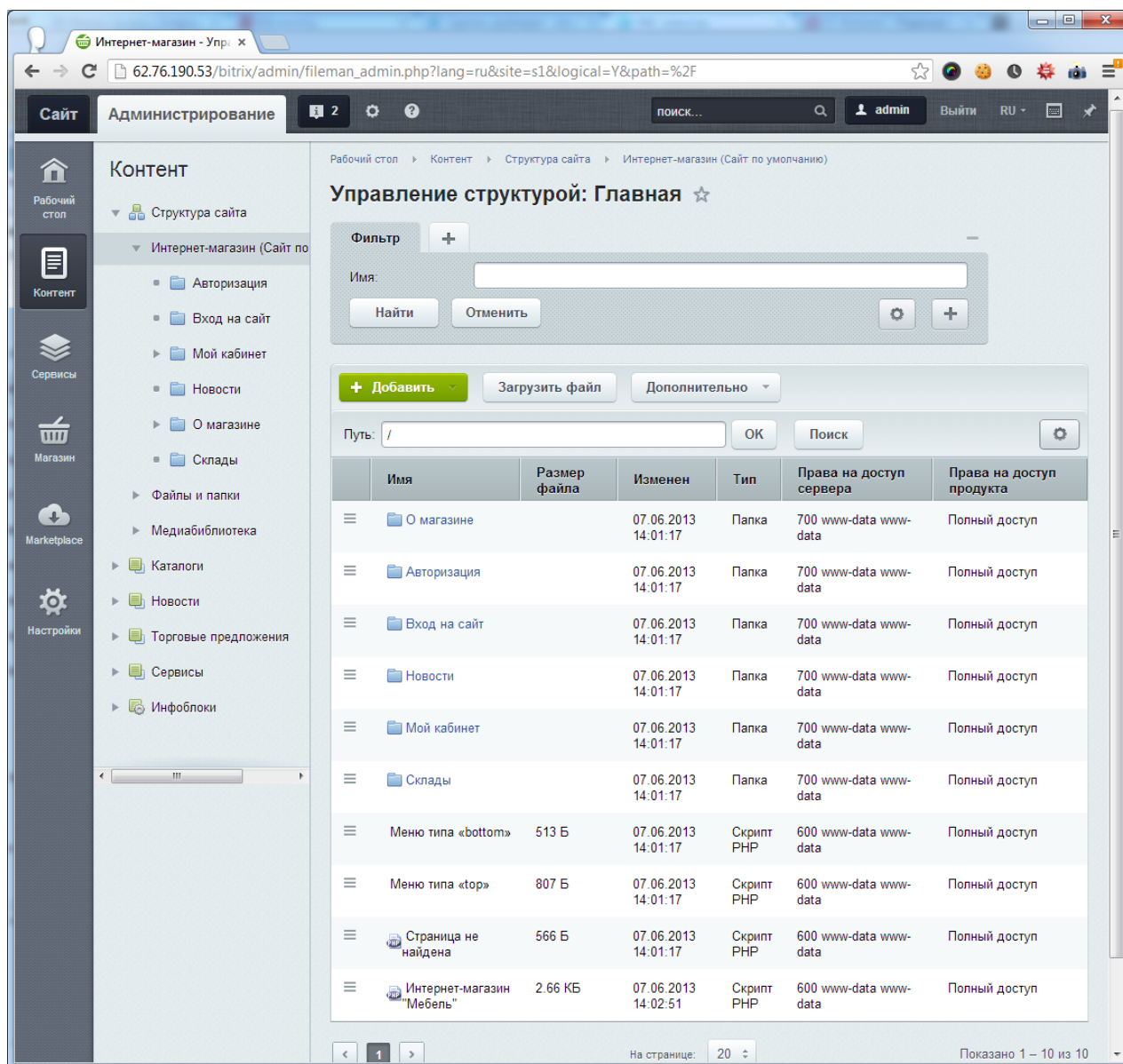
Рисунок 5. Добавление страницы.
